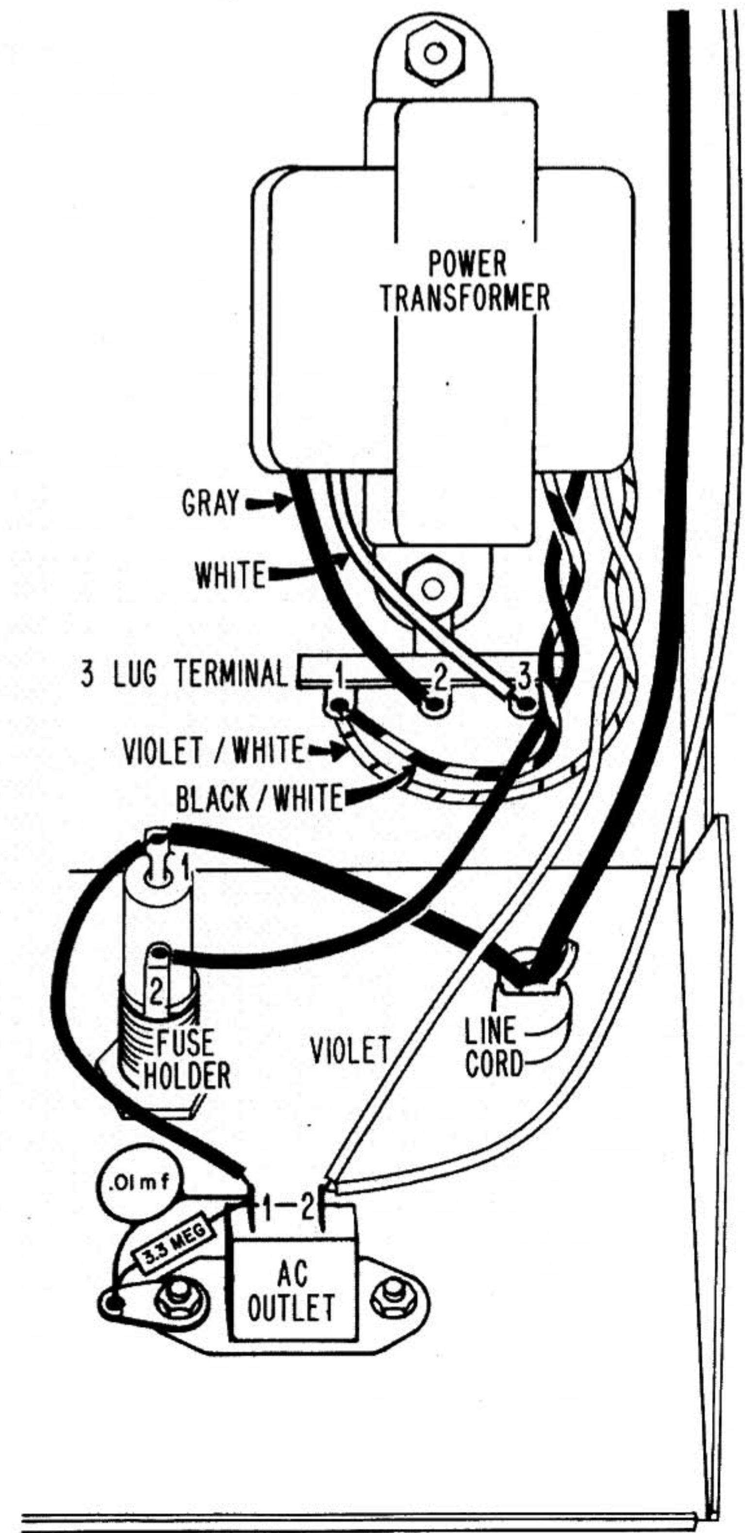
240 VOLT AC WIRING
